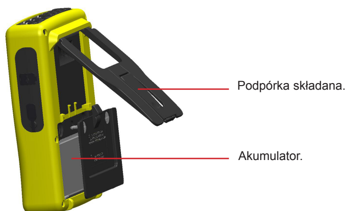
Rysunek 5: podpora i pokrywa zasobnika akumulatora
