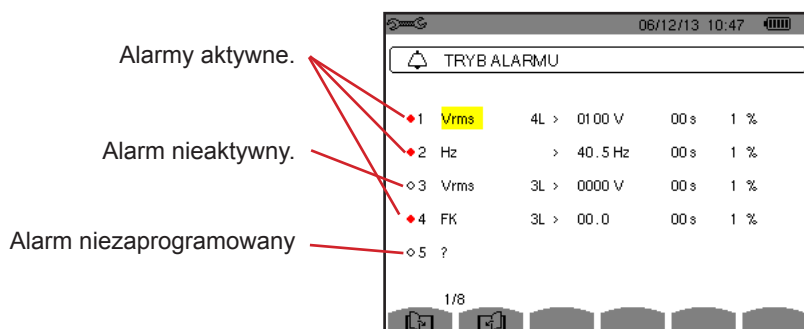
Rysunek 34: menu Trybu alarmu
