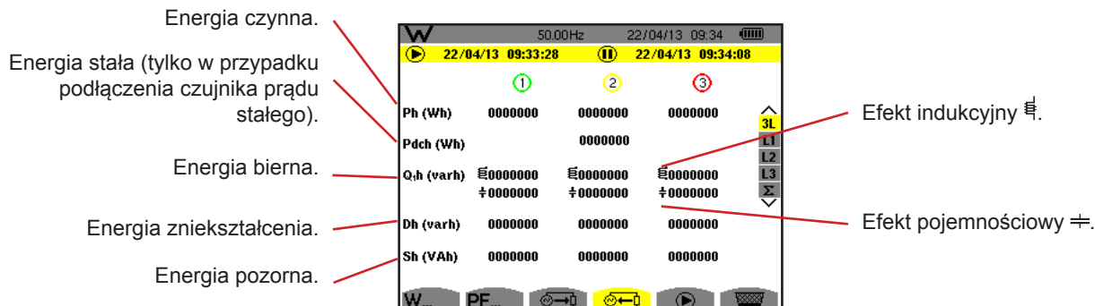
Rysunek 112: ekran wyświetlania energii generowanej w 3L
