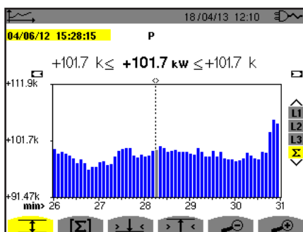
Rysunek 100: P (Σ) z MIN-AVG-MAX
