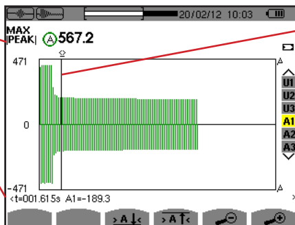
Rysunek 50: ekran wyświetlania PEAK w A1 dla podłączenia trójfazowego bez zera
