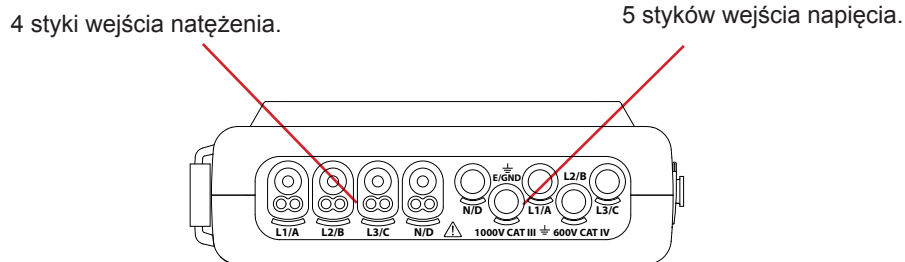
Rysunek 3: styki podłączeniowe
