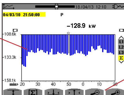
Rysunek 99: P (Σ) bez MIN-AVG-MAX
