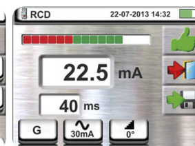
Ramp test wyniki RCD
