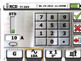
Wybór prądu wyzwalania na RCD z zewnętrznym transformatorem toroidalnym
