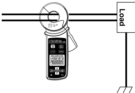
Instalacja 1-fazowa 2-przewodowa. W przypadku instalacji 3-przewodowej z przewodem neutralnym należy zacisnąć cęgi na wszystkich trzech przewodach.
