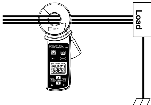
Instalacja 3-fazowa 3-przewodowa. W przypadku instalacji 3-fazowej 4-przewodowej z przewodem neutralnym należy zacisnąć cęgi na wszystkich czterech przewodach.
